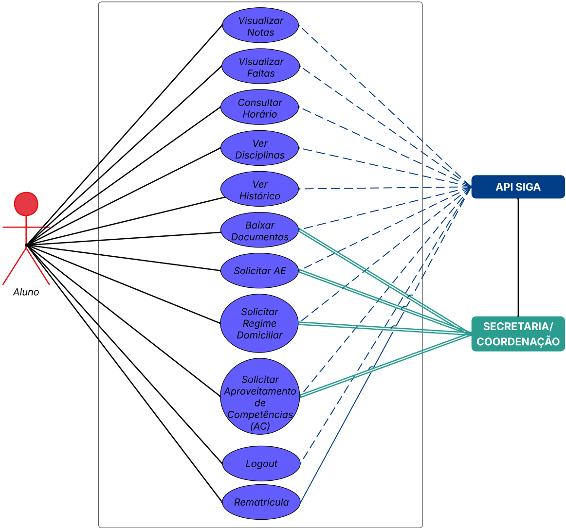
Diagrama de caso de uso - SIGA
